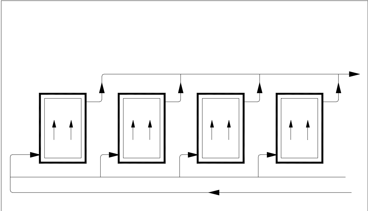
FIG. 15 CONEXIONADO DE CAPTADORES EN PARALELO
