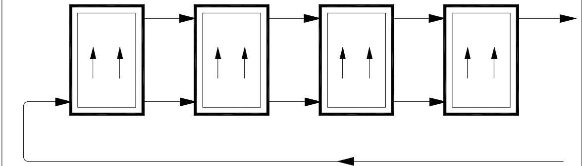
FIG. 16 CONEXIONADO DE CAPTADORES EN PARALELO
